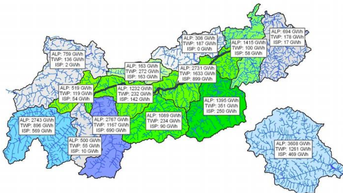
Abbildung 16: regionale Wasserkraftpotentiale ab 2MW Einzelleistung (Quelle: Wasserkraft in Tirol – Potenzialstudie 2011)
