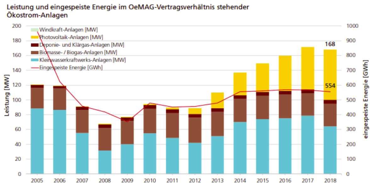
Abbildung 9: Leistung und eingespeiste Energie im ÖMAG-Vertragsverhältnis stehender Ökostrom-Anlagen in Tirol 21
