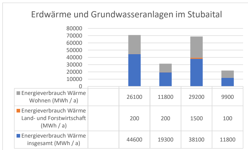
Abbildung 13: Erdwärme und Grundwasseranlagen im Stubaital 29
