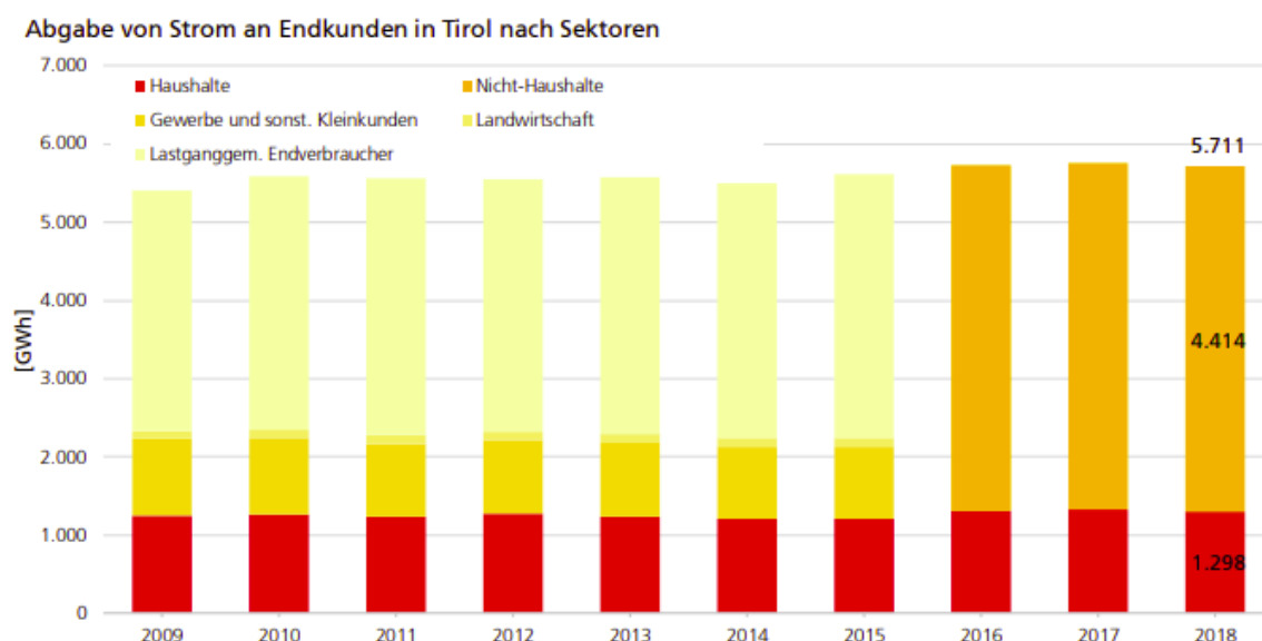
Abbildung 6: Stromverbräuche nach Sektoren des gesamten Bundeslandes Tirol 13
