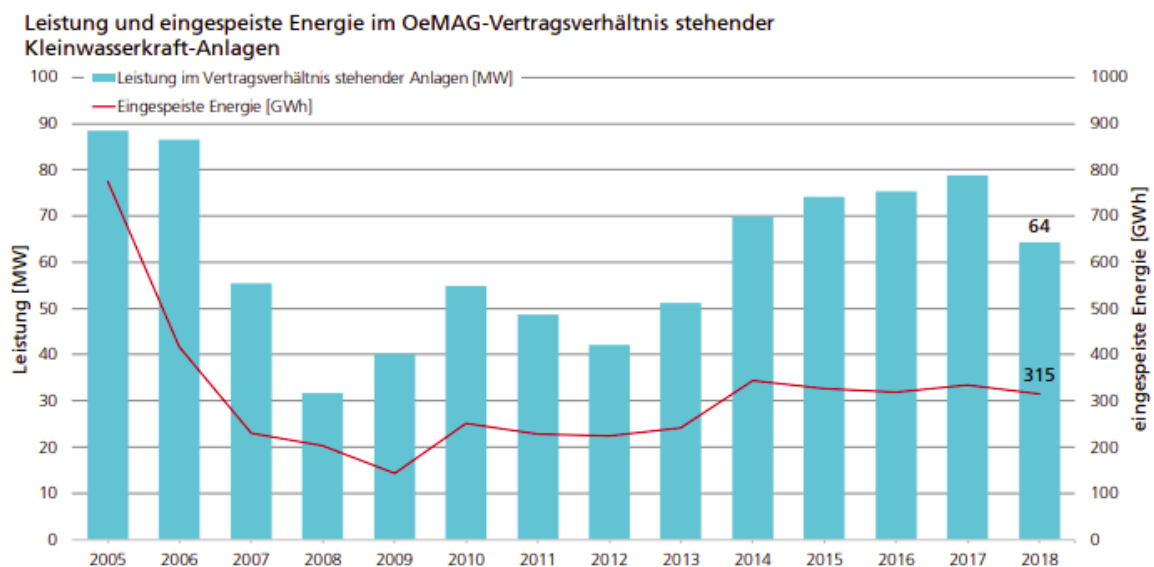
Abbildung 12: Leistung und eingespeiste Energie im OeMAG-Vertragsverhältnis stehender Kleinwasserkraft-Anlagen (Quelle: Energiemonitoring Tirol 2019)
