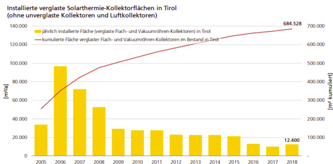
Abbildung 11: Installierte verglaste Solarthermie-Kollektorflächen in Tirol (Quelle: Energiemonitoring Tirol 2019)
