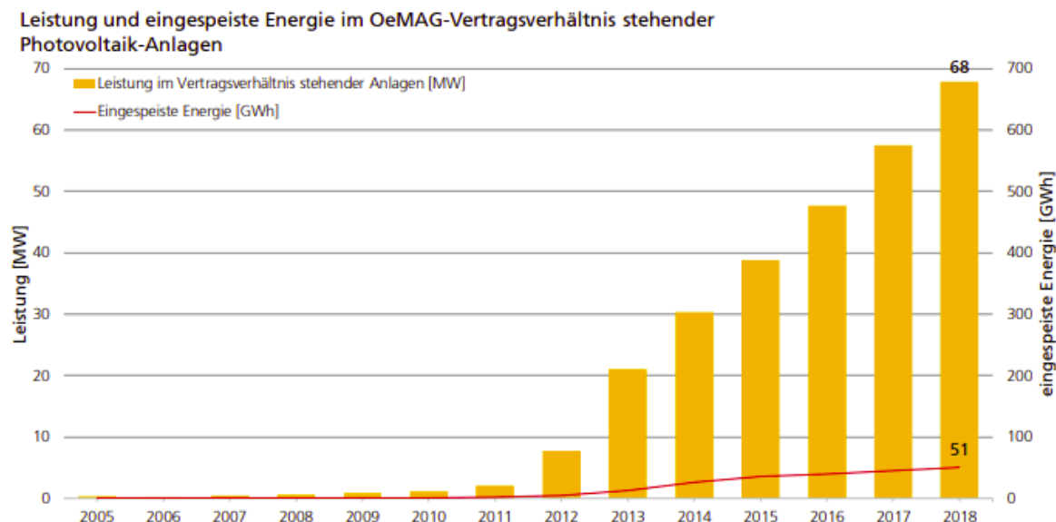
Abbildung 10: Leistung und eingespeiste Energie im ÖMAG-Vertragsverhältnis stehender PV-Anlagen im Jahr 2018 22
